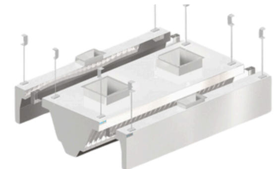
Coifa Lavadora
