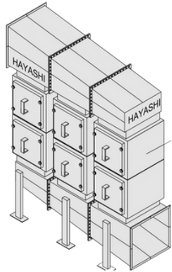
Gabinete de Precipitador Eletrostático ESP
