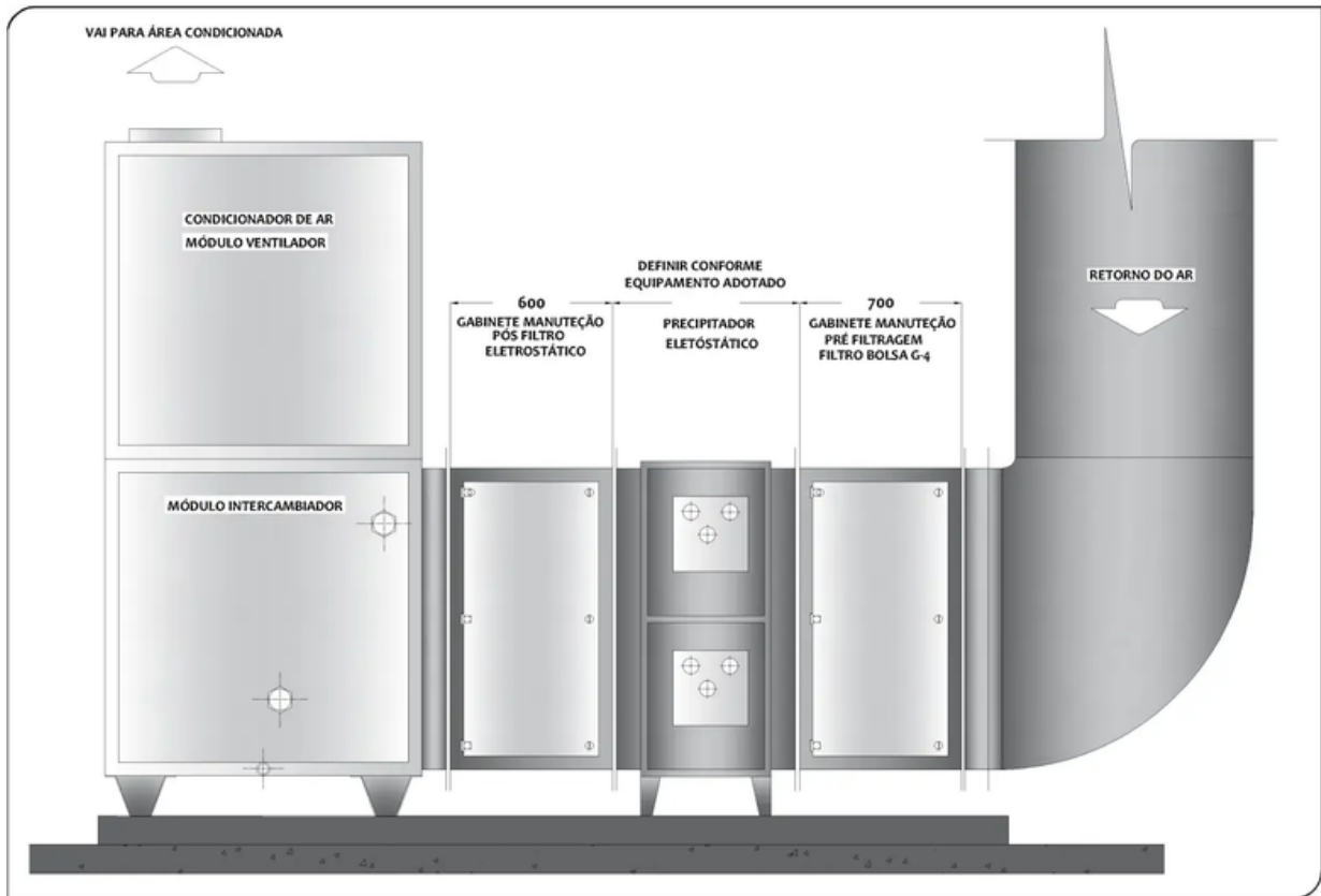
ELEVAÇÃO FRONTAL - SEM ESCALA
